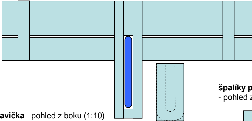
Středová lavička - pohled ze spodu (1:10)
